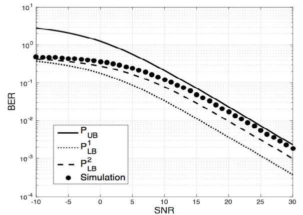
그림 1. QPSK가 적용된 물리계층 네트워크 코딩의 BER 성능
